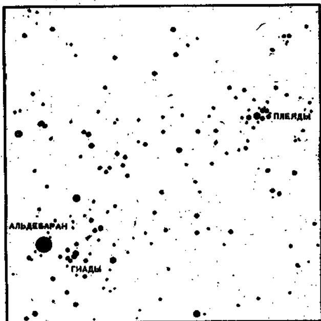
Рис. 52. Гиады и Плеяды в созвездии Тельца.
