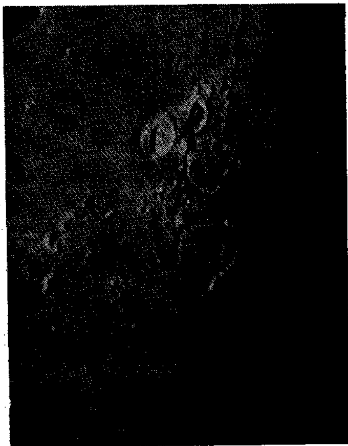
Рис. 98. Кратеры Аристарх, Геродот и долина Шретера.
