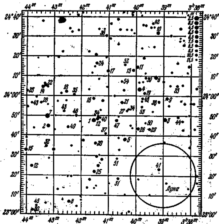
Рис. 50. Вид Плеяд в телескоп (кружком обозначены размеры лунного диска): 1 — Альциона, 2 — Атлас, 3 — Электра, 4 — Майя, 5 — Мерона, 6 — Тайгета, 7 — Плейона, 9 — Целена, 11 — Астеропа.
