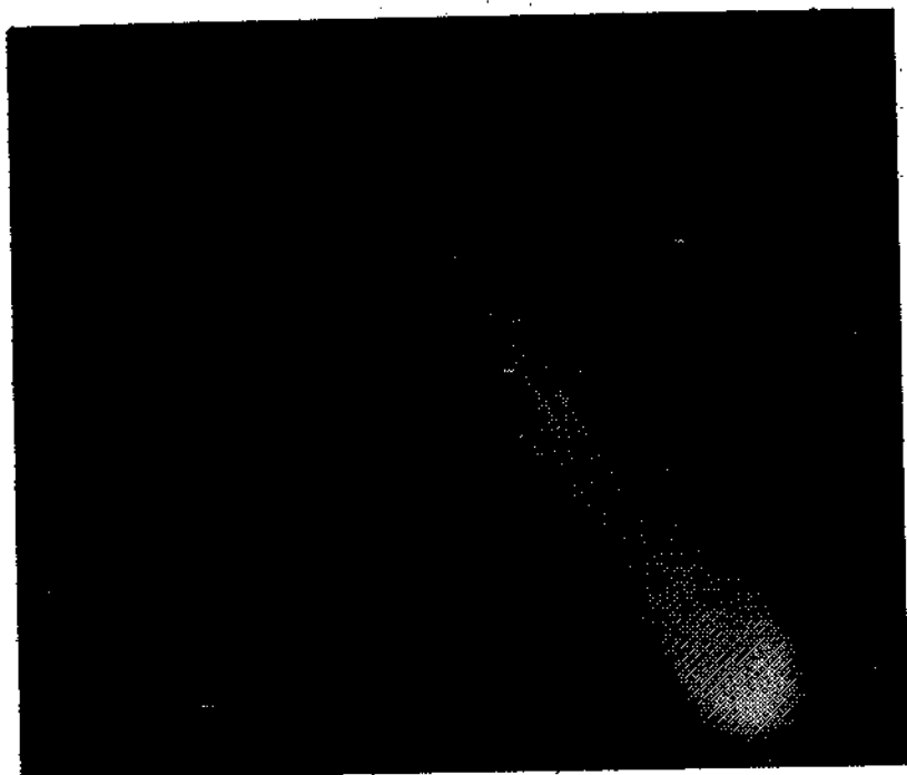
Рис. 74. Фотография кометы.
