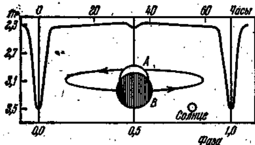
Рис. 41. Схема изменения блеска Алголя. вен периоду изменения блеска. Тем самым было
