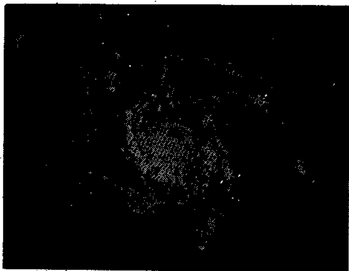
Рис. 33. Галактика М 101.
