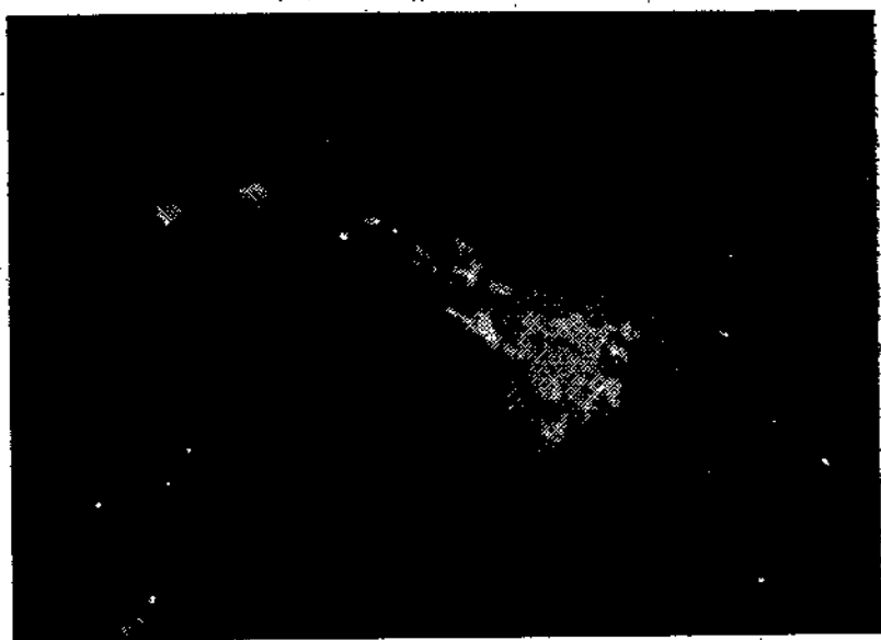
Рис. 71. Малое Магелланово Облако.
