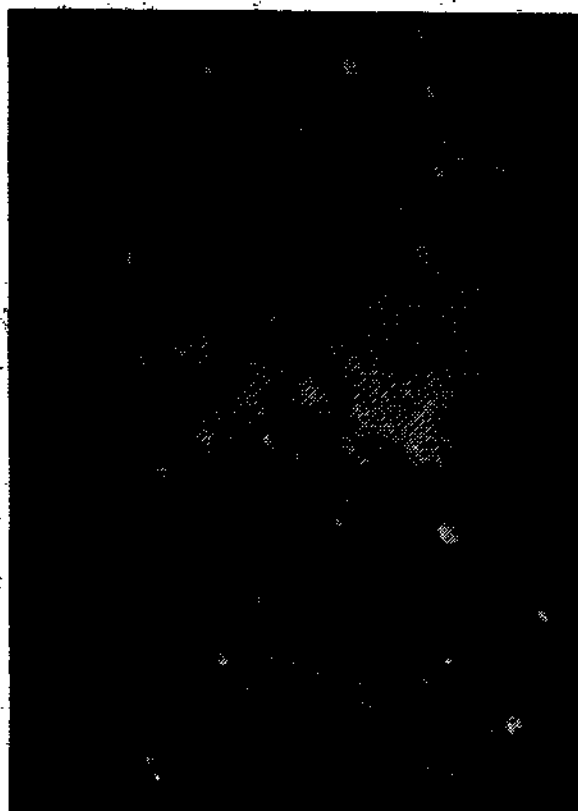
Рис. 66. Планетарная туманность в созвездии Лисички.
