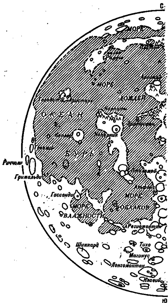
Рис. 79. Схематическая карта
