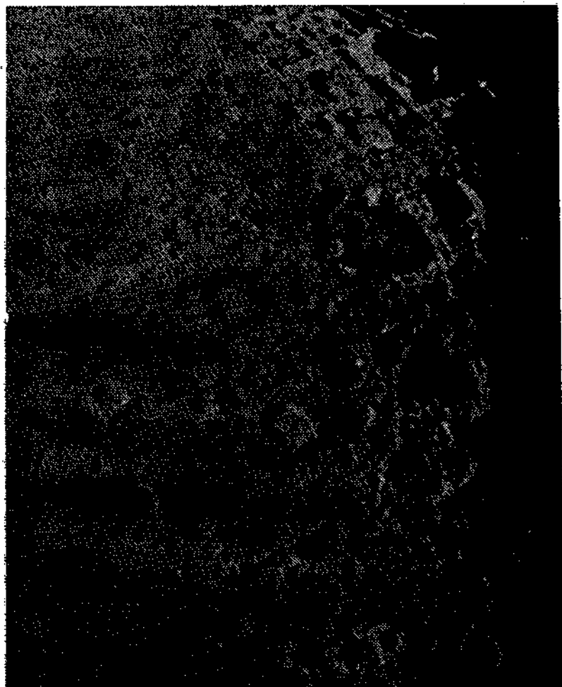
Рис. 80. Типичный лунный рельеф (область вблизи кратера Клавий).
