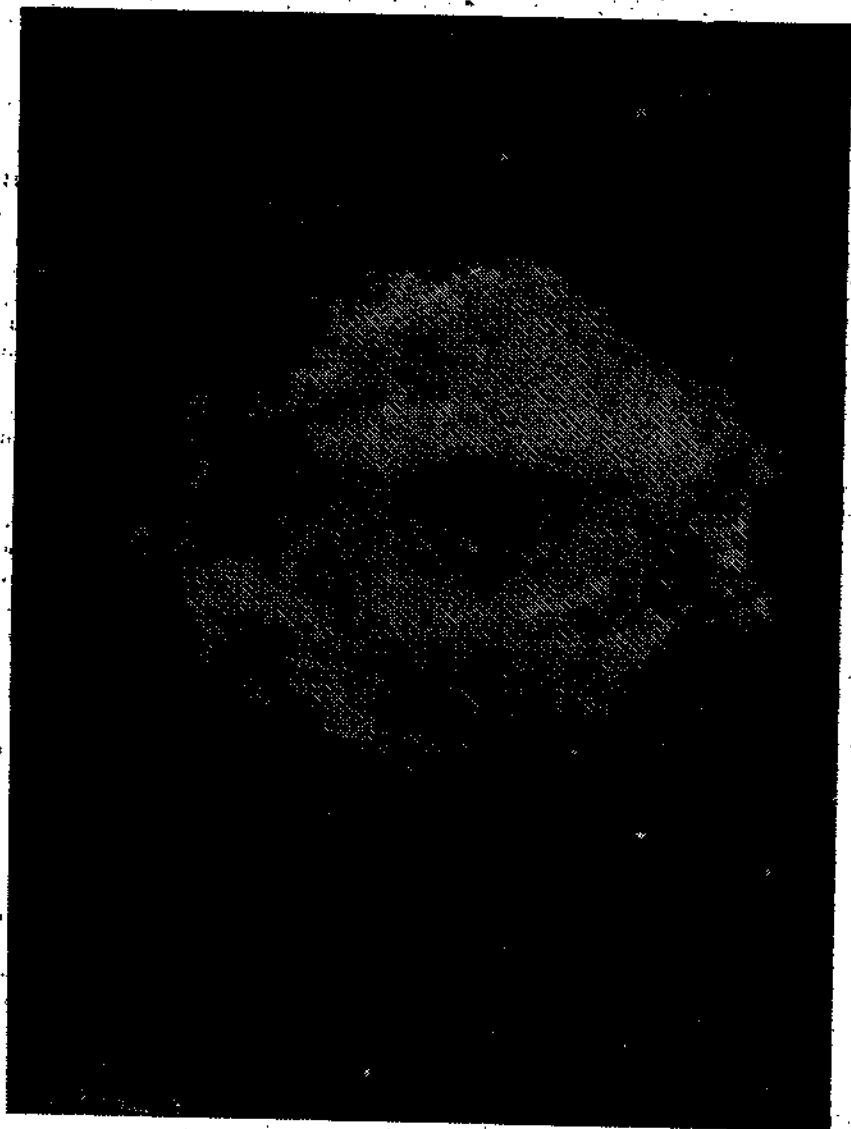
Рис. 57. Туманность «Розетка».
