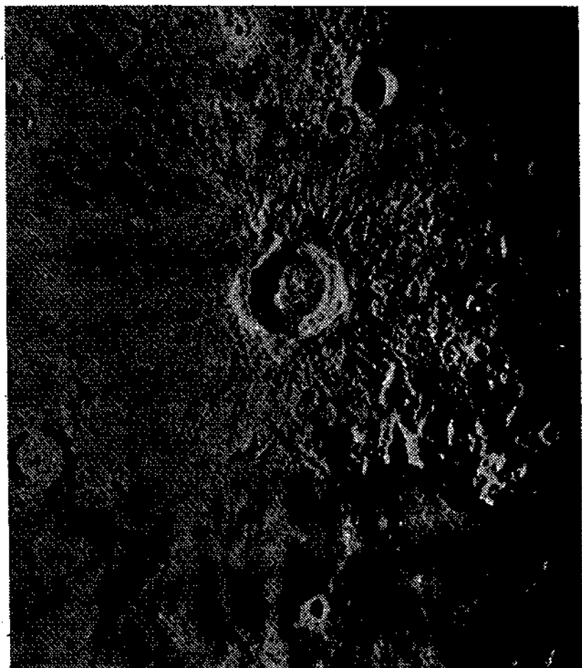
Рис. 92. Кратер Коперник и его окрестности.
