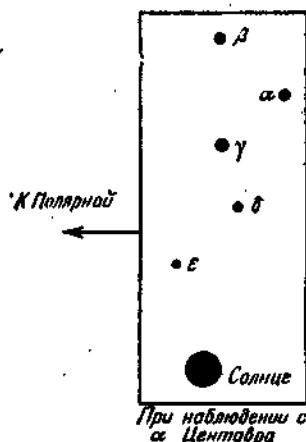
Рис. 73. Вид Солнца с \alpha Центавра.
