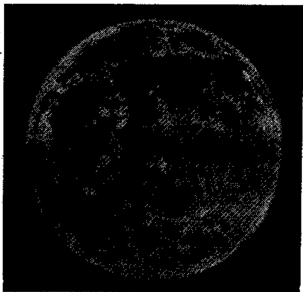
Рис. 77. Фотография полной Луны.
