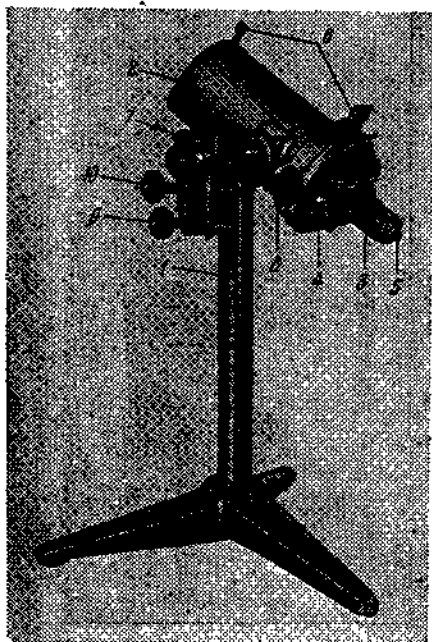
Рис. 17. Школьный менисковый телескоп. 1 — штатив, 2 — труба телескопа, 3 — окуляр с увеличением 25, 4 — окуляр с увеличением 70, 5 — зенитная призма, 6 — визиры для наведения на избранный объект, 7—10 — винты зажима и винты тонкой наводки прибора.
