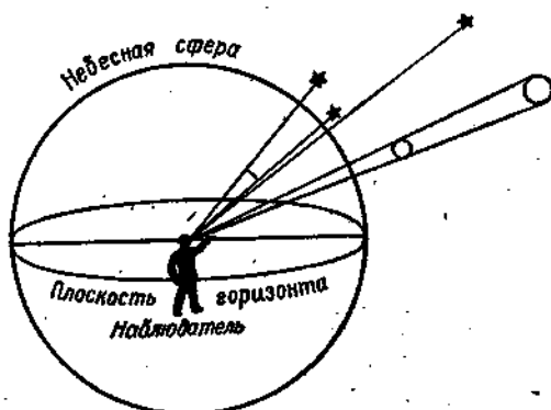
Рис. 19. Небесная сфера.
