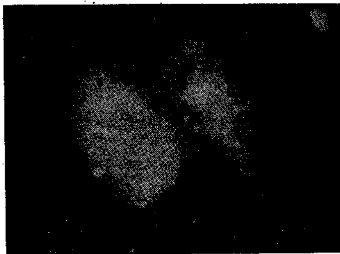
Рис. 68. Фотография в инфракрасных лучах части галактического ядра.
