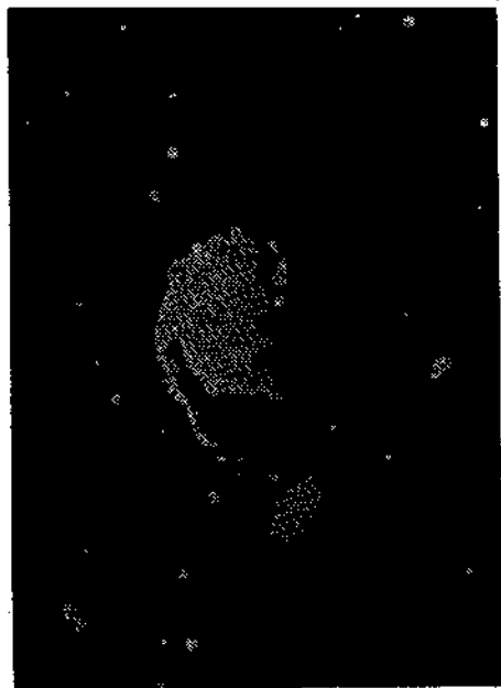
Рис. 59. «Двойник» галактики М 51.
