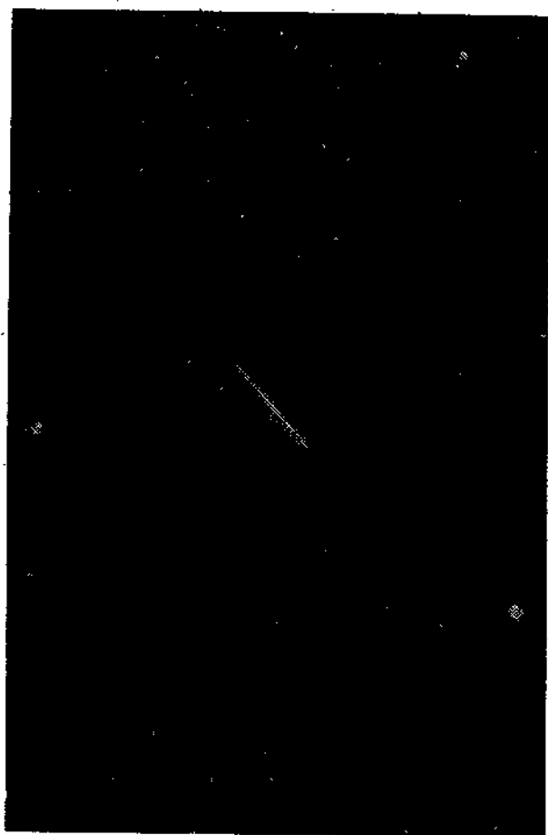
Рис. 75. Болид.
