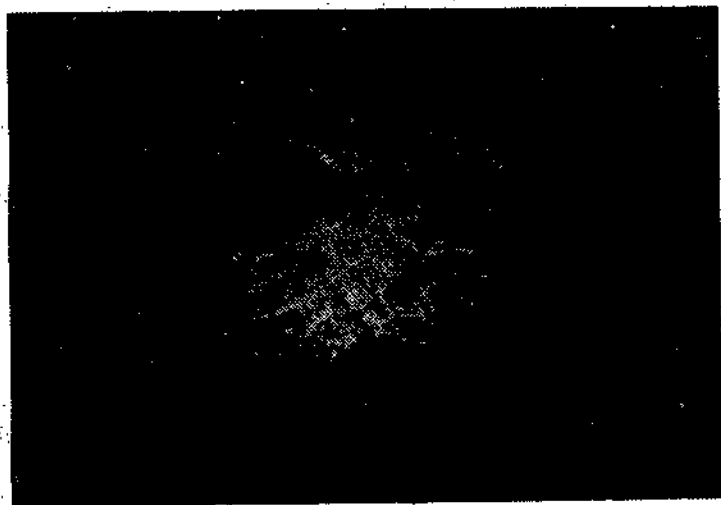
Рис. 54. Крабовидная туманность.
