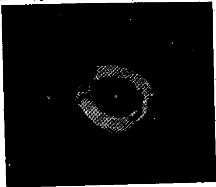
Рис. 61. Планетарная туманность в созвездии Лиры.
