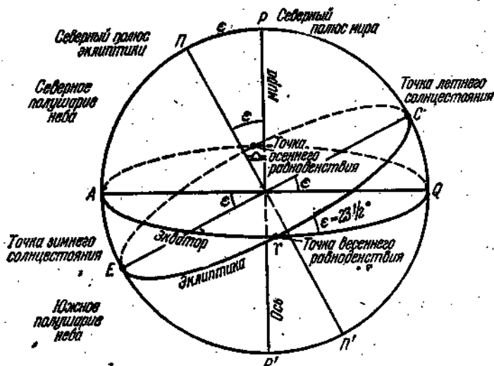
Рис. 26. Небесный экватор и эклиптика.
