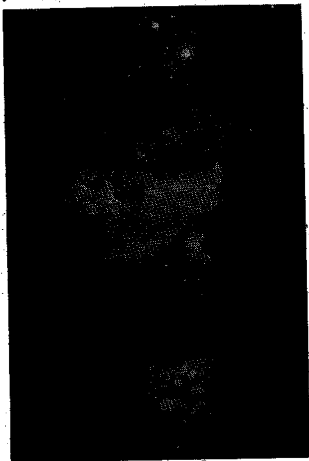
Рис. 49. Туманность Ориона.
