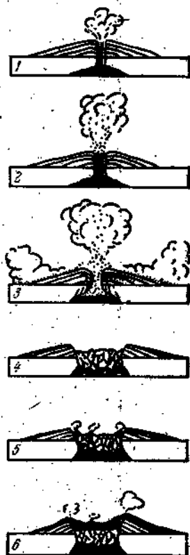
Рис. 84. Последовательные стадии образования кальдер.
